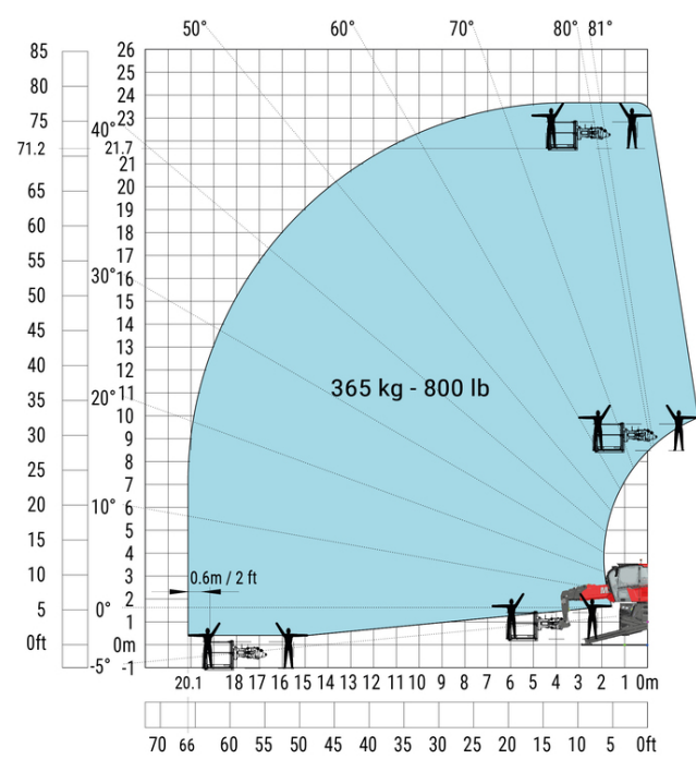
Rotazione su stabilizzatori con cestello da 365 kg
