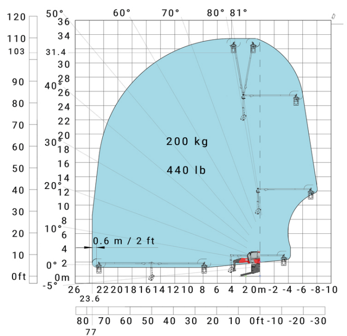
Rotazione su stabilizzatori con cestello 3D positivo
