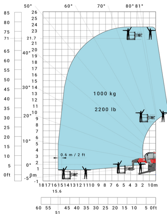
Rotazione su stabilizzatori con cestello da 1000 kg
