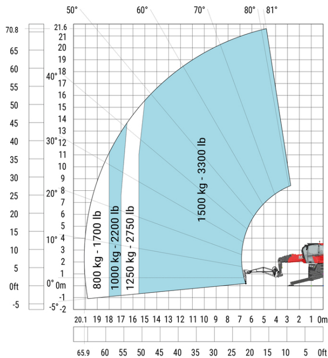
Rotazione su stabilizzatori con braccetto jib da 1500 kg
