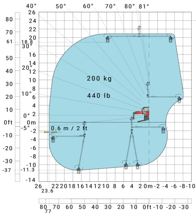
Rotazione su stabilizzatori con cestello 3D negativo
